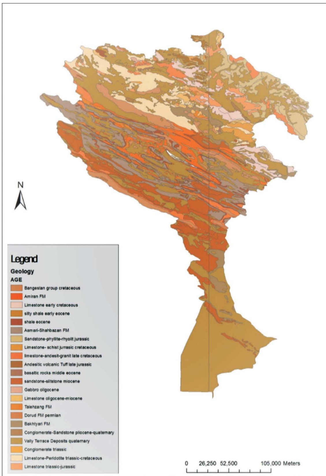
شکل ۳. نقشه زمین‌شناسی منطقه (استفاده از نقشه‌های سازمان زمین‌شناسی و به کارگیری آن در GIS)
