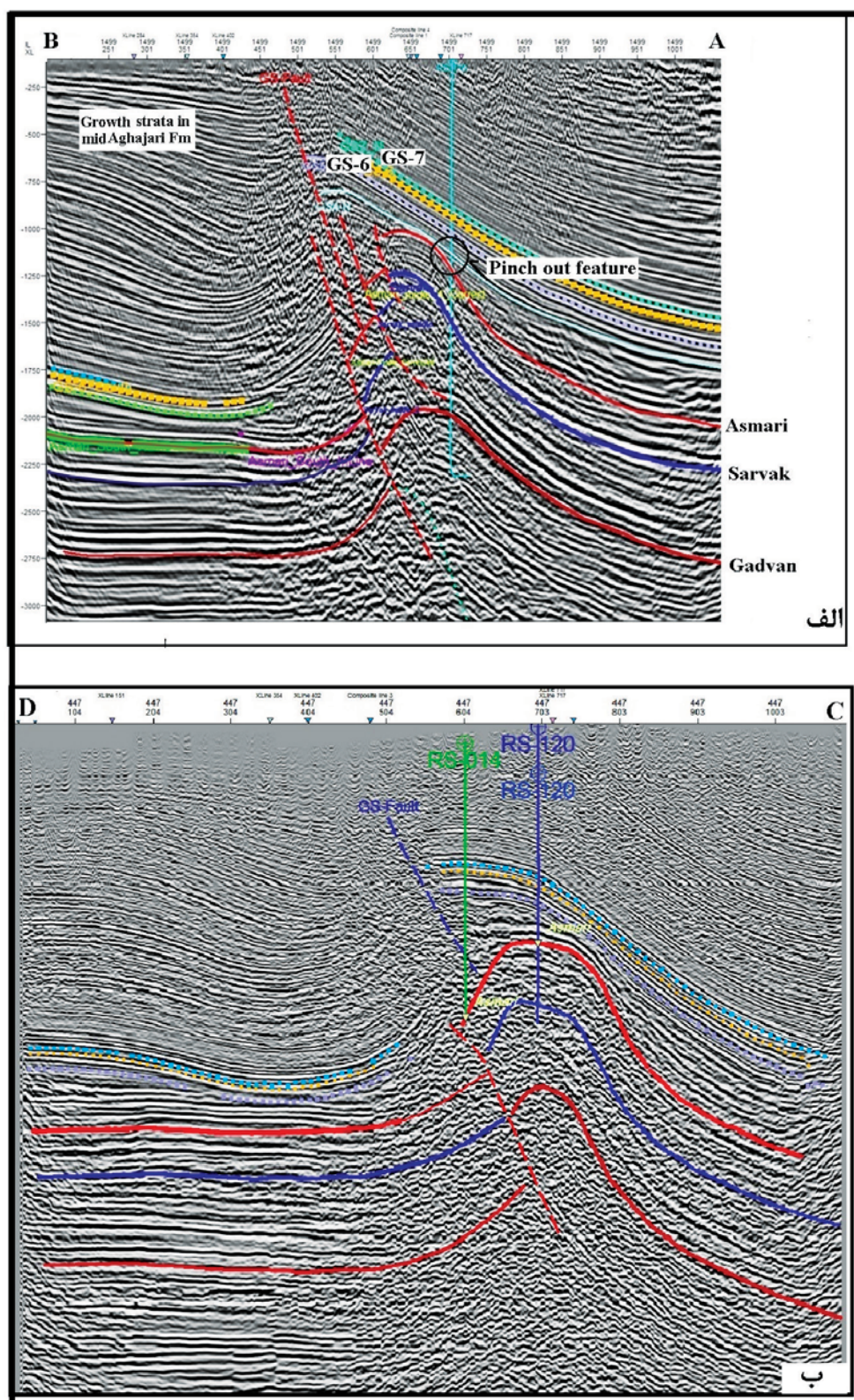
شکل ۴. الف و ب) نیمرخ‌های لرزه‌ای AB و CD به ترتیب در بخش شرقی و غربی تأقدیس رگ سفید: یک راندگی با عمق زیاد در یال جنوب غربی مشاهده می‌شود و با ادامه دگرریختی یک راندگی بالایی با ریشه در سازند گچساران به سطح رسیده است. همچنین اثر مهاجرت و انتشار راندگی‌ها در فرودبواره راندگی‌های قبلی مشهود است
