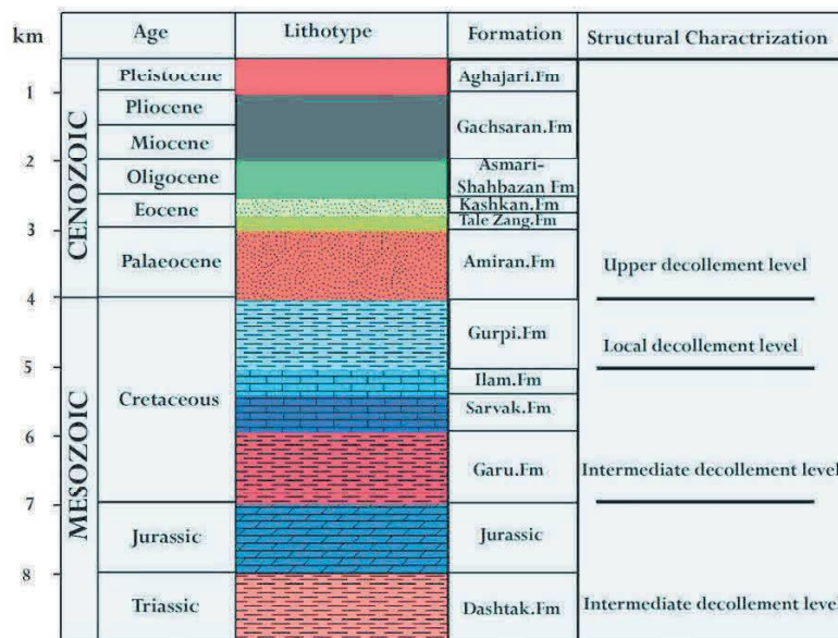
شکل ۳. ستون چینه‌شناسی سازندهای مزوزویک و سنوزویک در بخش مرکزی زیرپهنه لرستان که سطوح جدایشی و ضخامت رخساره‌های رسوبی را نشان می‌دهد
