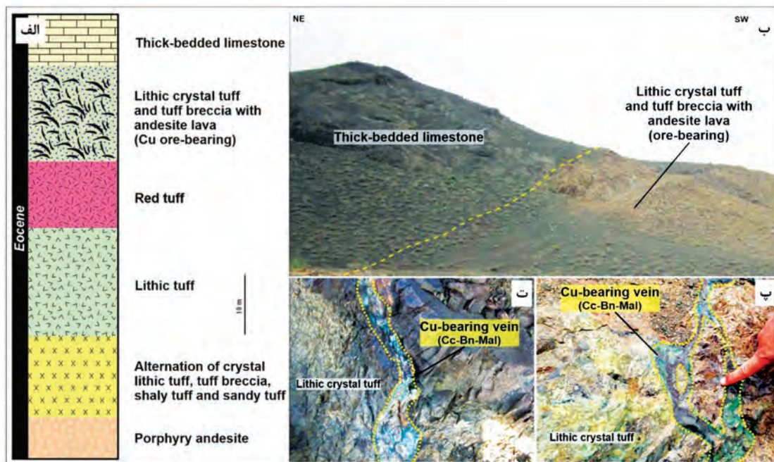
شکل ۴. الف) ستون چینه‌شناسی توالی آتشفشانی-رسوبی ائوسن در کانسار کهک و موقعیت کان‌زایی چینه‌کران مانتو در آن (دید به سمت جنوب-شرق)، ب) دورنمایی از رخنمون واحدهای لیتیک کریستال توف و سنگ‌آهک در محدوده معدنی کهک، پ و ت) نمایی از رخنمون کان‌زایی رگه-رگچه‌ای مس در واحد کریستال لیتیک توف در کانسار کهک (کالکوسیت: Cc، بورنیت: Bn، مالاکیت: Mal) (نشانه‌ها برگرفته از Whitney and Evans, 2010)
