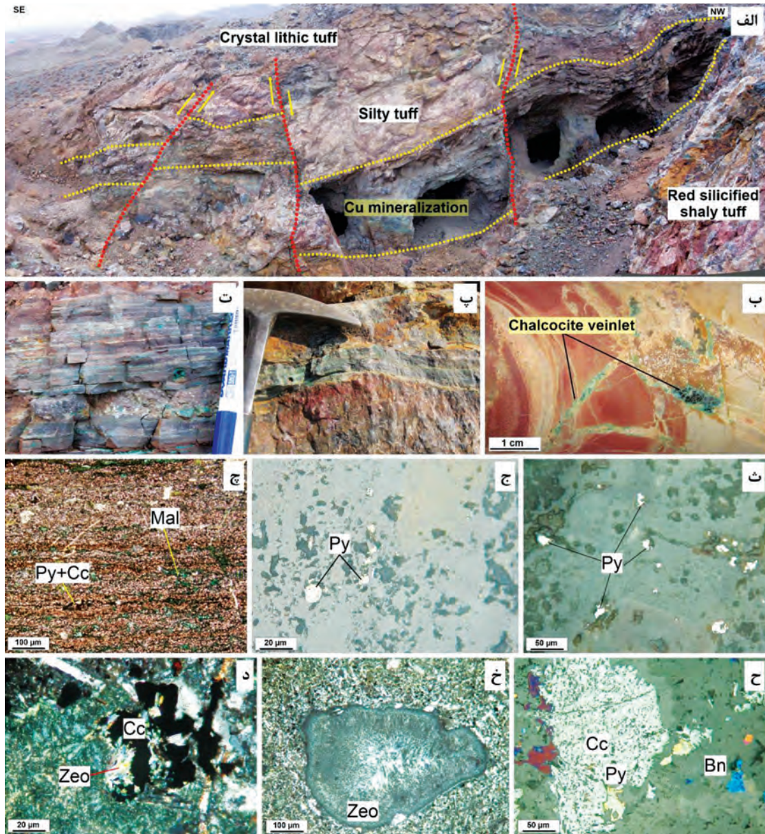
شکل ۹. الف) دورنمایی از رخداد کانه‌زایی مس چینه‌کران در واحد توف سیلنتی و فعالیت‌های معدنی ششادای صورت گرفته در آن، ب) تصویر نمونه دستی بافت رگه-رگچه‌های کالکوسیت که لایه‌بندی سنگ میزبان را قطع کرده است، پ و ت) کانه‌زایی مس که به صورت هم‌روند با لامیناسیون سنگ میزبان رخ داده است، ث) تصویر میکروسکوپی از پیریت دانه‌پراکنده در متن سنگ میزبان توف سیلنتی، ج) تصویر میکروسکوپی از پیریت‌های فرامیوئیدال، چ) تصویر میکروسکوپی (نور عبوری) توف سیلنتی و بافت دانه‌پراکنده پیریت و سولفیدهای مس در آن، ح) تصویر میکروسکوپی کانسنگ رگه-رگچه‌ای که در آن کالکوسیت در حال جانشینی پیریت است، خ) تصویر میکروسکوپی حفرات پر شده سنگ میزبان از کانی زئولیت، د) تشکیل زئولیت و کالکوسیت به صورت پرکننده فضای خالی در متن سنگ میزبان (کالکوسیت: Cc، بورنیت: Bn، پیریت: Py، مالاکیت: Mal، زئولیت: Zeo) (نشانه‌ها برگرفته از Whitney and Evans, 2010)
