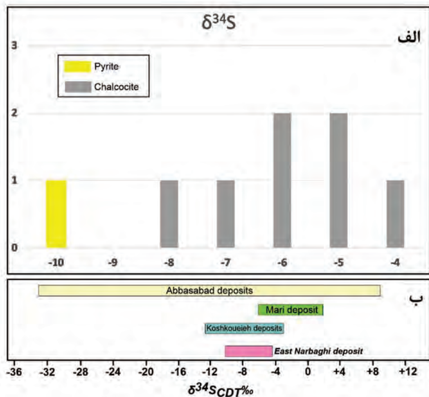
شکل ۱۰. الف) نمودار ستونی نسبت ایزوتوپی گوگرد در نمونه‌های سولفیدی کانسار نارباغی شرقی، ب) نمودار مقایسه‌ای مقادیر \delta^{34}\text{S} در کانسارهای مس مانتو با سن سنگ میزبان ائوسن در ایران (صالحی و رسا، ۱۳۹۴؛ ابولی‌پور، ۱۳۹۱؛ Maghfouri et al., 2017).
