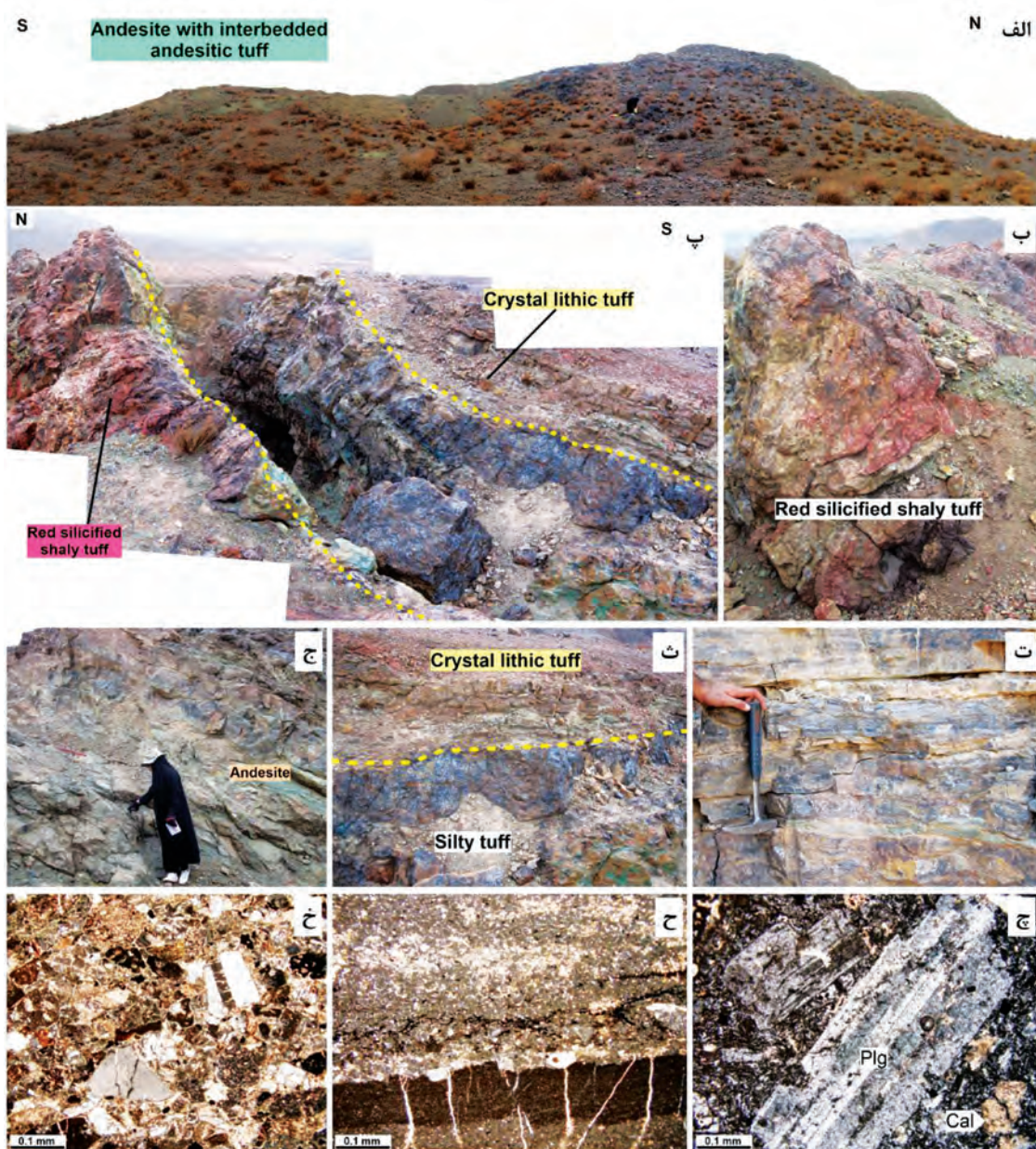
شکل ۸. الف) دورنمایی از رخنمون واحد آندزیتی با میان لایه‌های توف آندزیتی در بخش شمالی محدوده معدنی نارباغی شرقی (دید به سمت غرب)، ب) رخنمون واحد توف شیلی قرمز رنگ سیلیسی شده (کمبراییین ماده معدنی)، پ) رخنمون واحد توف سیلیتی میزبان کانه‌زایی و واحدهای کمربالایی و کمربالایی آن (دید به سمت شرق)، ت: نمایی نزدیک از رخنمون واحد توف سیلیتی میزبان کانه‌زایی، ث) همبری واحدهای توف سیلیتی (میزبان کانه‌زایی) و کریستال لیتیک توف (کمبرالایی کانه‌زایی)، ج) رخنمون واحد آندزیتی، چ) تصویر میکروسکوپی میان لایه‌های آندزیتی واحد میزبان کانه‌زایی، ح) تصویر میکروسکوپی توف سیلیتی میزبان کانه‌زایی، خ) تصویر میکروسکوپی میان لایه‌های توف برش واحد میزبان کانه‌زایی مس در کانسار نارباغی شرقی (پلاژیوکلاز: Plg، کلسیت: Cal) (نشانه‌ها برگرفته از Whitney and Evans, 2010)
