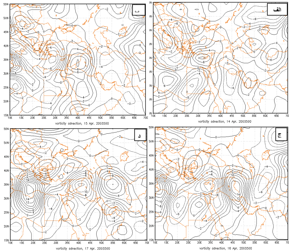
شکل ۷: میدان فرارفت تاوایی تراز ۵۰۰ هکتوپاسکال (حسب بر ثانیه بر متر) برای ساعت ۰۰۰۰ UTC روزهای ۱۴ تا ۱۷ آوریل ۲۰۰۳ به ترتیب از الف تا د مأخذ: نگارندگان، ۱۳۹۲
