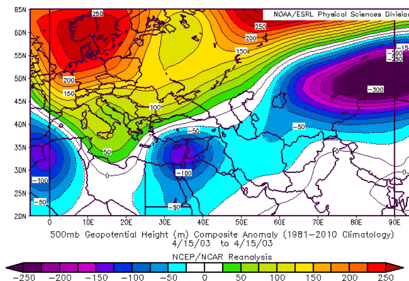
شکل ۵: بی‌هنجاری ارتفاع تراز ۵۰۰ هکتوپاسکال نسبت به میانگین بلندمدت آن در روز ۱۵ آوریل ۲۰۰۳ مأخذ: نگارندگان، ۱۳۹۲
