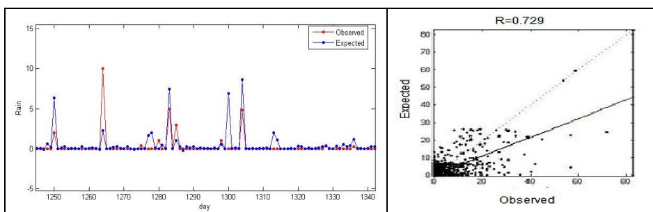
شکل ۴ - مقایسه نتایج شبکه عصبی (Expected) و داده‌های واقعی (Observed) در مدل MLP33 بافت و
