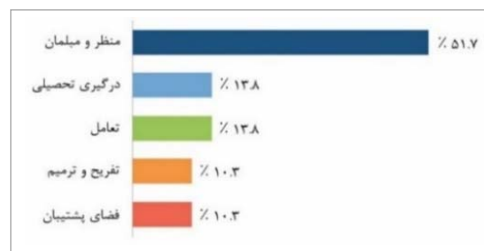
تصویر ۶. نمودار فراوانی عوامل مرتبط با رضایتمندی دانشجویان در محوطه روبه‌روی کتابخانه (نگارندگان)
