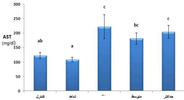
نمودار ۲. مقایسه آنزیم آسپارات امینوترانسفراز در گروه‌های مورد بررسی
