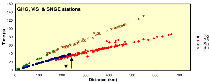
شکل ۱۶. نمودار زمان-مسافت موج‌های P و S به روش دوایستگاهی در امتداد مسیرهای قلقزی، ویس و سندج شکل ۱
