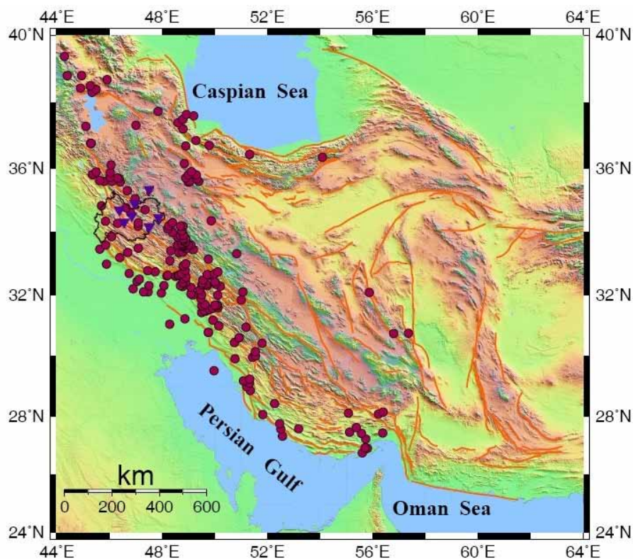
شکل ۵. نقشه موقعیت زمین‌لرزه‌های انتخاب شده همراه با ایستگاه‌های لرزه‌نگاری غرب ایران. برای ترسیم منحنی‌های زمان-مسافت در امتدادهای نشان داده شده در شکل ۱
