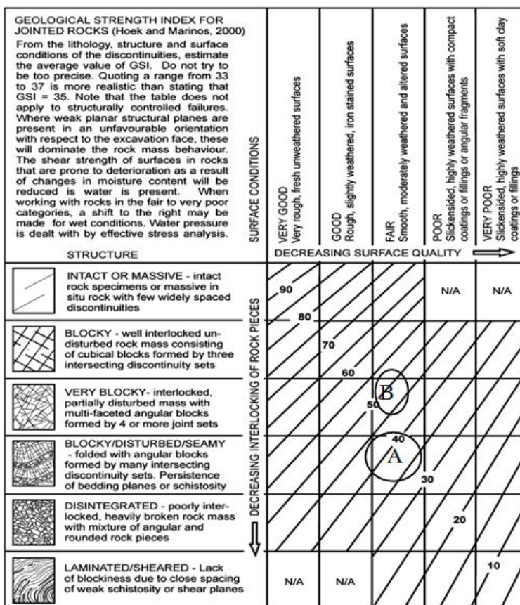
شکل ۵. تعیین عدد GSI برای مصالح سازند گچساران
