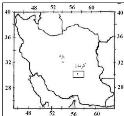
شکل ۱. موقعیت دشت کرمان-باغین در ایران
