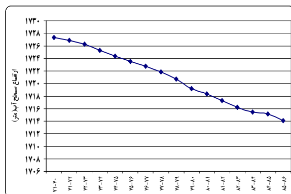
شکل ۶. هیدروگراف واحد ۱۶ ساله دشت کرمان- باغین
