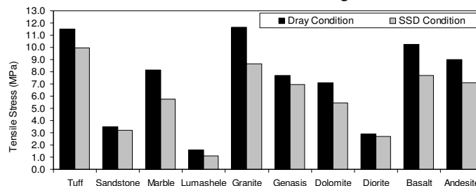
شکل ۶. نتایج آزمایش مقاومت کششی برزیلین
