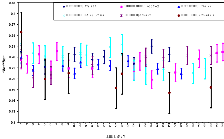
شکل ۴. تفاوت حد آستانه ارائه شده توسط برنامه و حد آستانهٔ بهینه برای نمونه‌های مختلف
