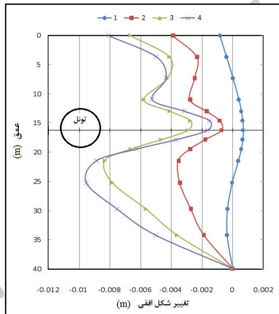
شکل ۱۱. جابه‌جایی‌های افقی خاک در راستای محور X : (۱) جبهه‌کار در فاصله ۱۰/۵ متری از محل بررسی، (۲) عبور ابتدای سپر، (۳) عبور انتهای سپر، (۴) جابه‌جایی نهایی
