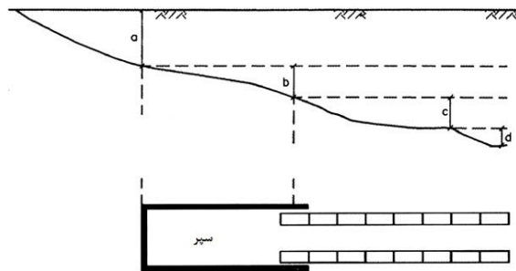
شکل ۳. مراحل نشست زمین ناشی
