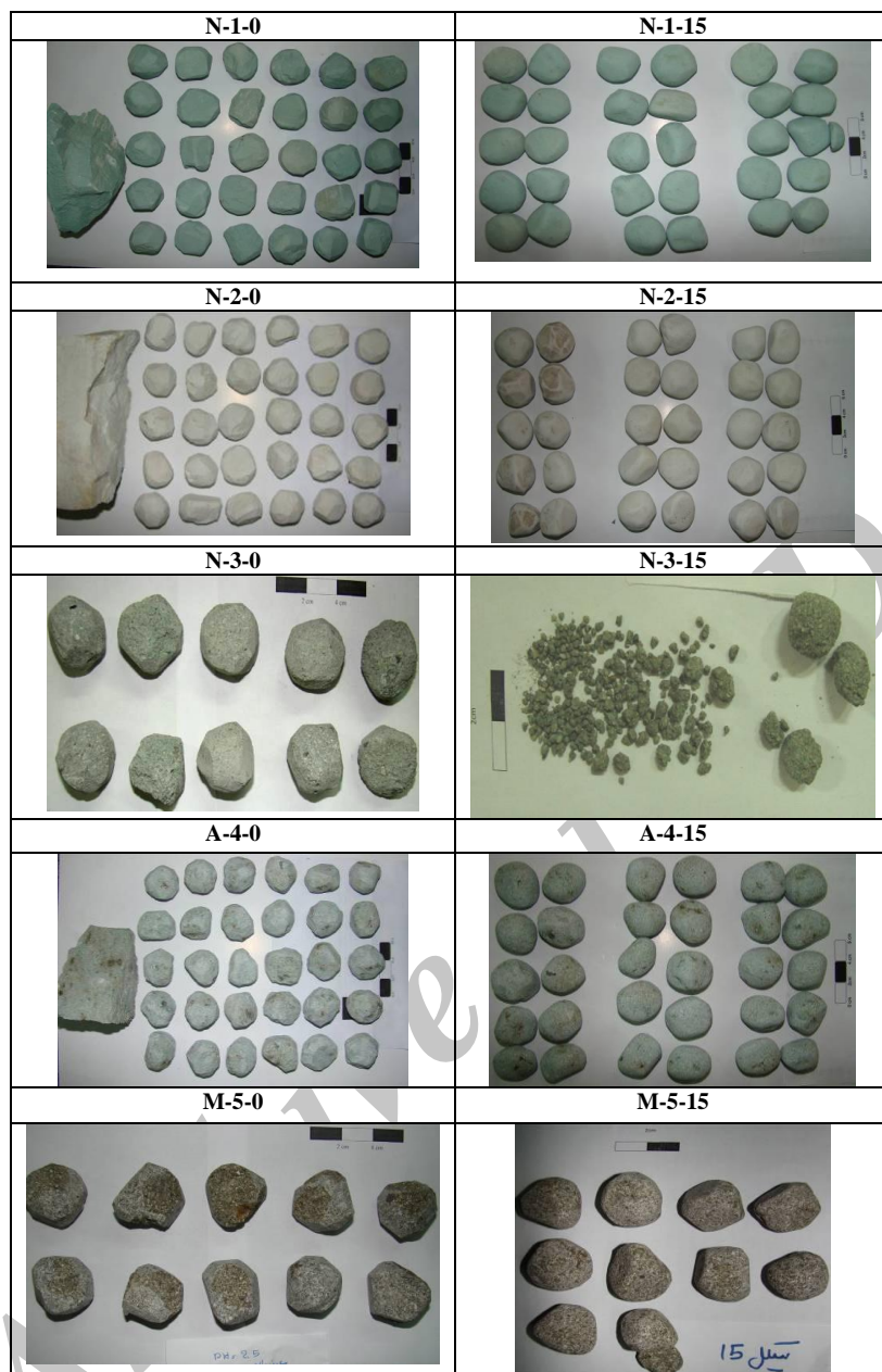
شکل ۶. تغییرات در شکل نمونه و اندازه نمونه‌های دوام بعد از ۱۵ سیکل از انجام آزمون دوام و وارفتگی در pH=2.5 ، کدهای بالای هر عکس نشان‌دهنده نوع سنگ (جدول ۱) و تعداد سیکل آزمون دوام است.
