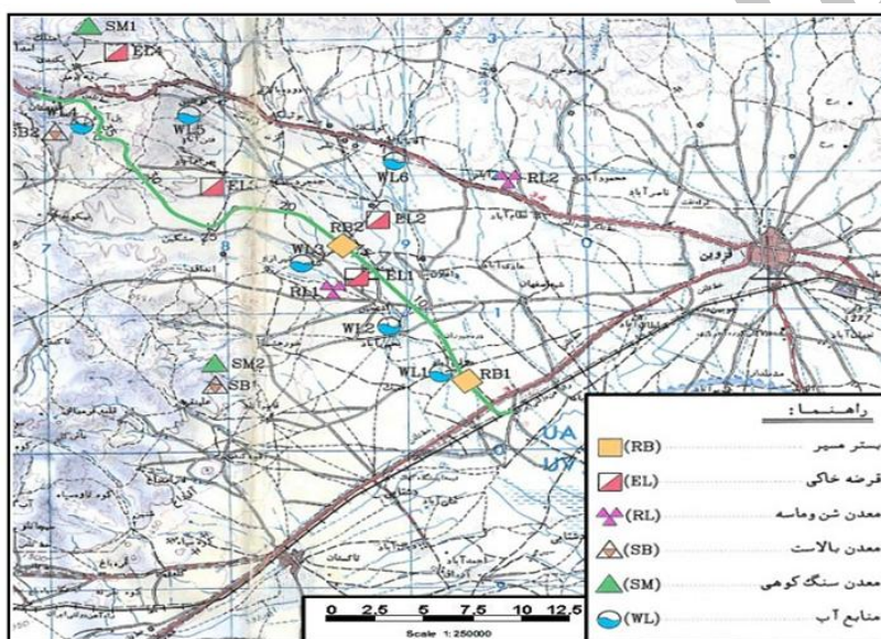
شکل ۱. موقعیت جغرافیایی تونل کوهین واقع در قطعه اول راه آهن قزوین - رشت - بندر انزلی به مقیاس (۱:۲۵۰۰۰۰)
