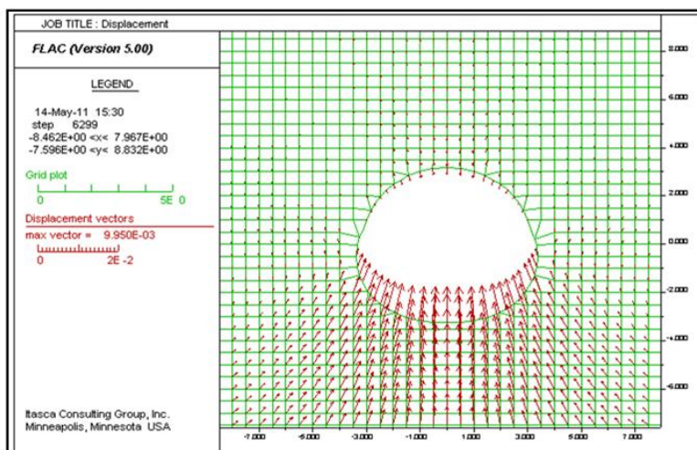
شکل ۹. بردارهای جابه‌جایی در اطراف تونل بعد از نصب سیستم نگه‌داری بنچینگ (مقطع
