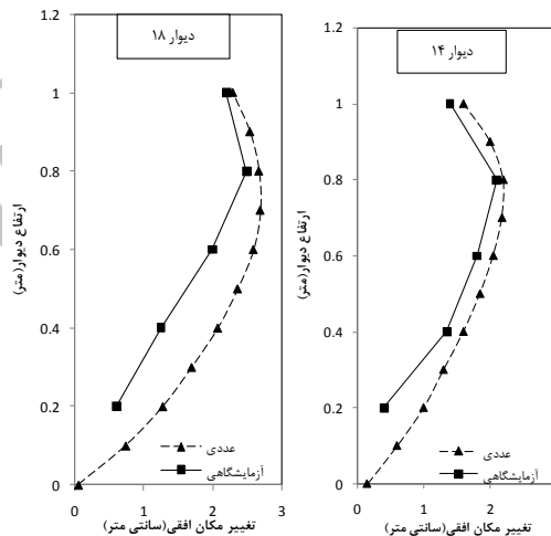
شکل ۵. مقایسه مقدار تغییر شکل نمای دیوار در پژوهش‌های آزمایشگاهی (صابر ماهانی ۱۳۸۷) و عددی برای مود شکم‌دادگی
