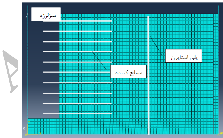
شکل ۳. اجزای مدل عددی ارائه شده در این تحقیق
