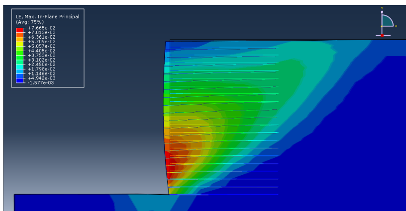
شکل ۱۰. نقاط پلاستیک در مود شکم‌دادگی
