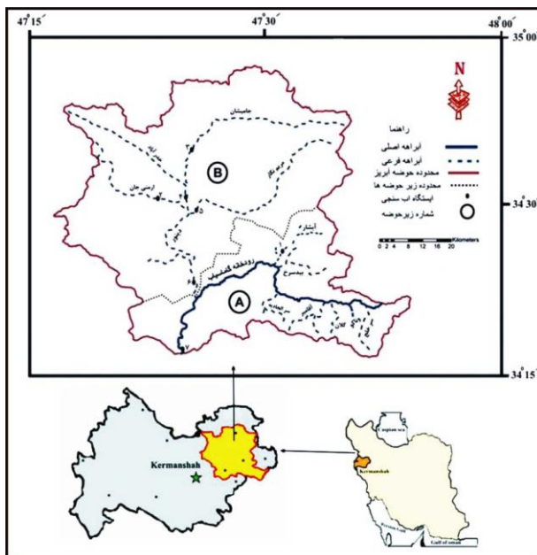
شکل ۳. موقعیت زیرحوزه‌ها و ایستگاه‌های آب‌سنجی در حوزه آبریز گاماسیاب پایین (ایستگاه‌های آب‌سنجی ۱. صحنه، ۲. خدرآباد، ۳. پیرسلمان، ۴. میانراهان، ۵. کله‌جوب، ۶. حیدرآباد، ۷. پل‌چهر) [۱۱]
