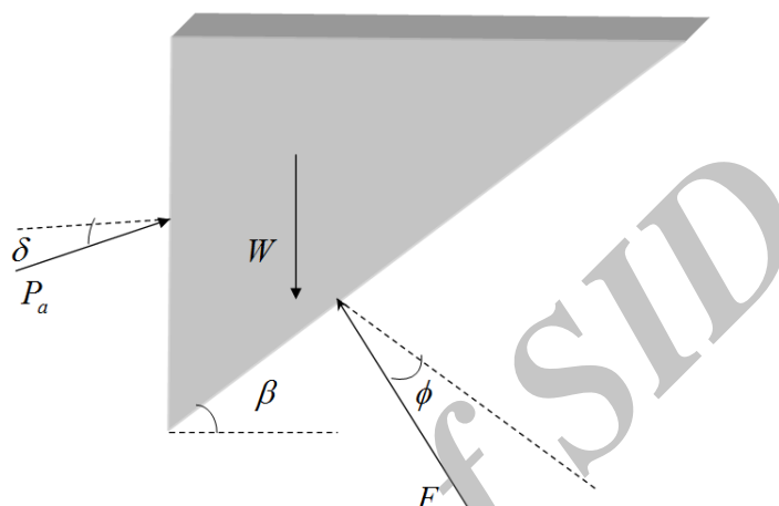
شکل ۳. تعادل ناحیه فعال ایجاد شده پشت دیوار حائل
