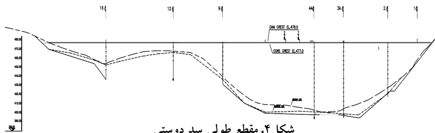
شکل ۴. مقطع طولی سد دوستی
