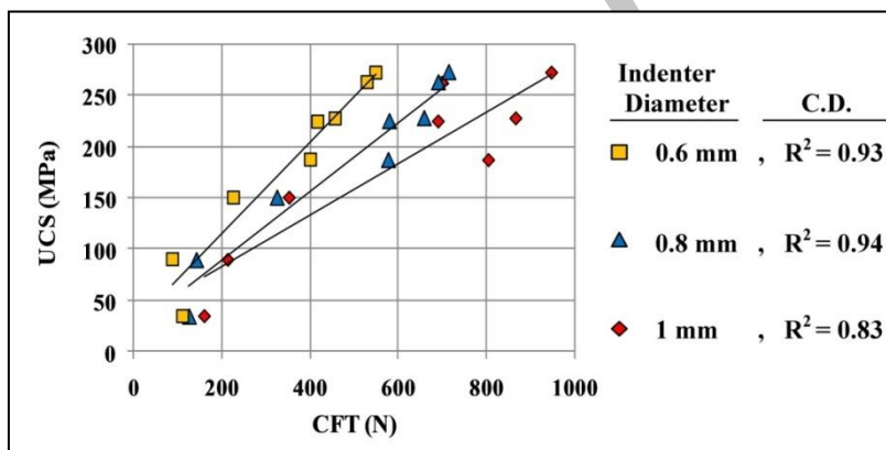
شکل ۷. هم‌بستگی CTF-UCS مربوط به خرده‌های سنگی ۳ میلی‌متری که با نفوذکننده‌های ۰/۶، ۰/۸ و ۱ میلی‌متری آزمایش شده‌اند.
