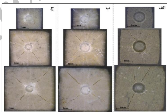
شکل ۴. ذرات خرده سنگی پس از آزمایش نفوذ. که با استفاده از نفوذکننده‌های مختلف (الف) ۱ میلی‌متری، ب) ۰/۸ میلی‌متری و ج) ۰/۶ میلی‌متری، تحت نفوذ قرار گرفته‌اند
