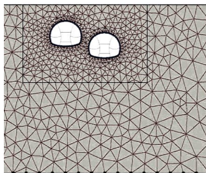
شکل ۱۰. مدل‌بندی المان محدود
