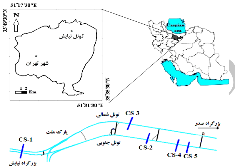
شکل ۱. موقعیت تونل نیایش و مقاطع بررسی شده در مسیر تونل
