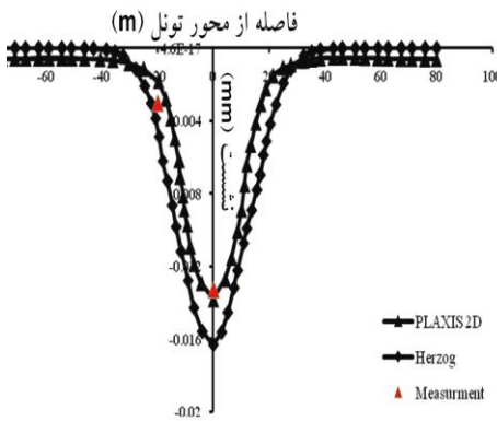
شکل ۱۵. الگوی نشست برای مقطع CS-5
