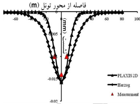
شکل ۱۲. الگوی نشست برای مقطع CS-2
