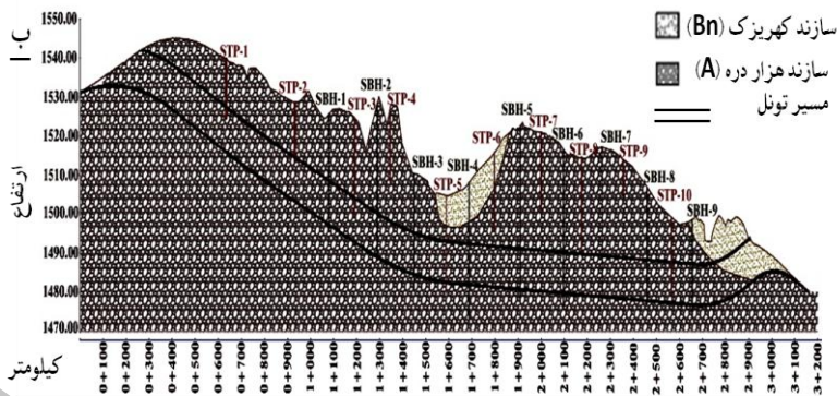
شکل ۲. مقاطع عرضی محدوده بررسی شده (الف: تونل شمالی، ب: تونل جنوبی) [۷]
