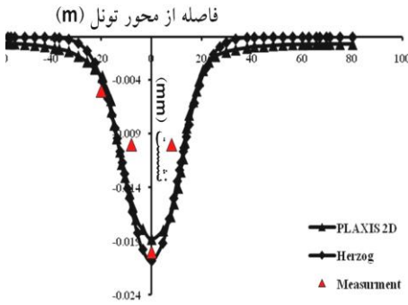
شکل ۱۳. الگوی نشست برای مقطع CS-3
