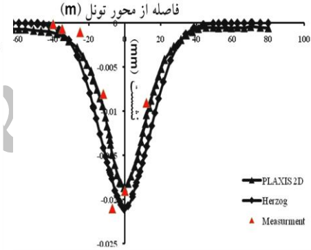
شکل ۱۴. الگوی نشست برای مقطع CS-4
