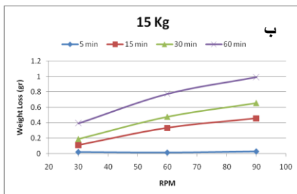
شکل ۱۲. میزان افت وزن تجمعی پیچ‌ها با تغییر در میزان سرعت چرخش برای سرباره‌های الف (۵، ب) ۱۵ و ج) ۲۰ کیلوگرم.
