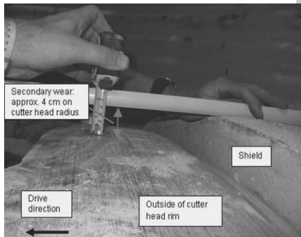
شکل ۳. سایش ثانویه زیاد در دیواره خارجی کله حفار یک ماشین EPB با قطر حفاری ۴/۷ متر [۷]
