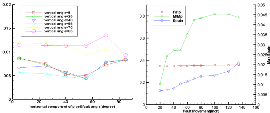
شکل ۸. تغییرات کرنش بیشینه، لنگر خمشی و نیروی محوری بر حسب میزان جابه‌جایی گسل شکل ۹. تغییرات کرنش بیشینه بر حسب مؤلفه افقی و قائم زاویه عبوری از گسل
