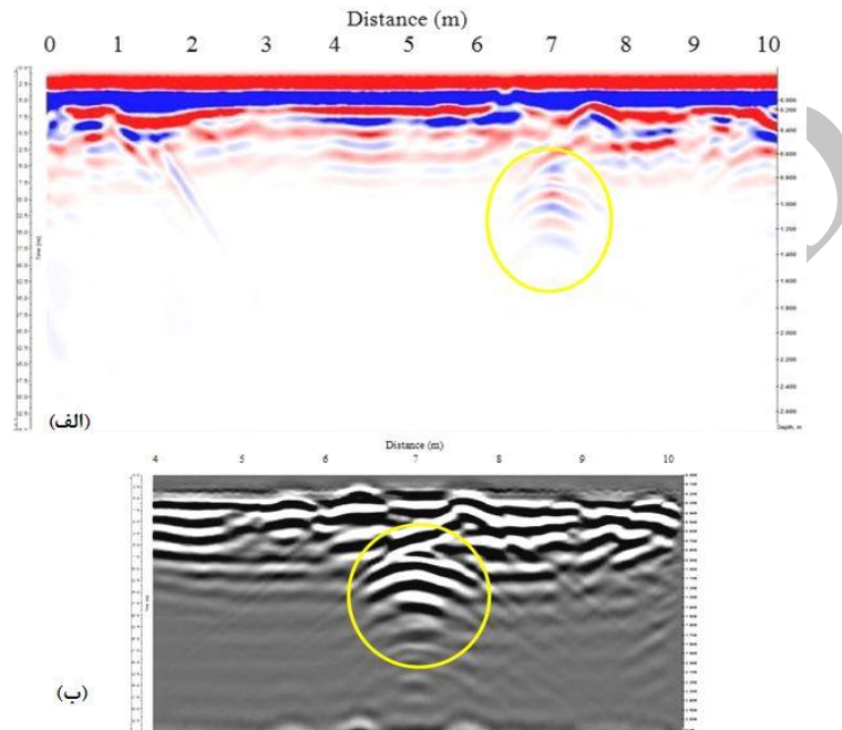
شکل ۱۱: الف) نگاهت راداری داده های خام، ب) بخشی از نگاهت راداری بعد از اعمال مراحل پردازشی مورد نیاز
