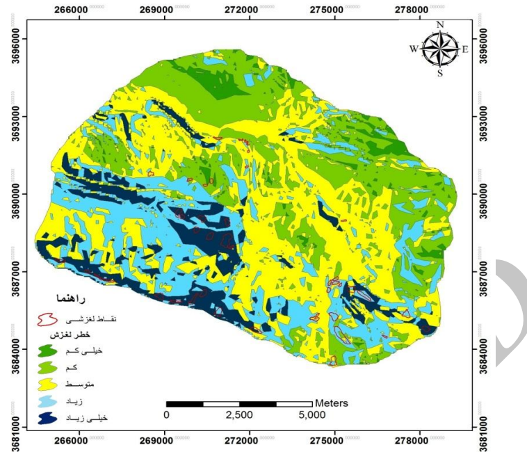
شکل ۱۴. نقشه پهنه‌بندی خطر زمین‌لغزش در حوضه کاکاشرف با استفاده از منطق فازی (عمل‌گر جمع فازی)
