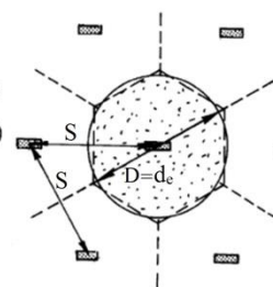
شکل ۱. چاه های زهکش [۲]
