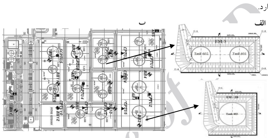
شکل ۷. الف) پلان موقعیت خاکریزهای EM-3 و EM-2B. ب) محل گمانه‌های ناحیه دو و سه ژئوتکنیکی
