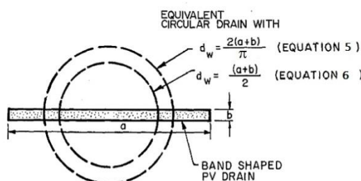
شکل ۲. قطر معادل زهکش نواری [۲]
