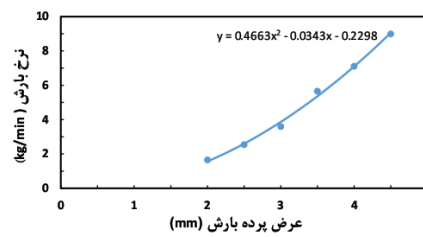
شکل ۱۰. اثر عرض پرده بارش (W) بر نرخ بارش
