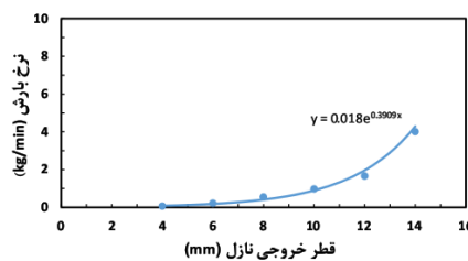
شکل ۱۱. اثر قطر خروجی نازل بر نرخ بارش
