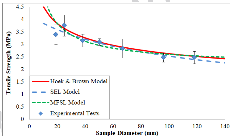
شکل ۱۰. مقایسه نتایج آزمایشگاهی با مدل‌های هوک و براون، SEL و MFSL
