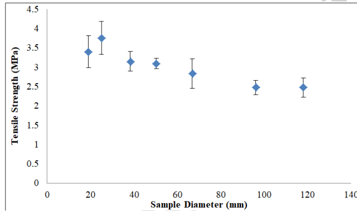
شکل ۸. مقایسه نتایج آزمون‌های برزیلی در قطرهای مختلف
