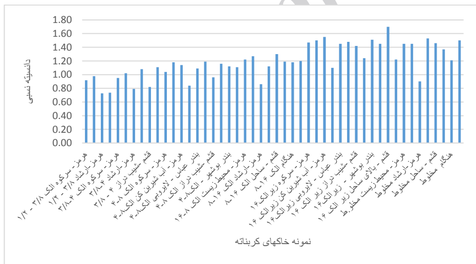
شکل ۵. نمایش دانسیته نسبی ۰.۵۰ نمونه خاک‌های کربناته
