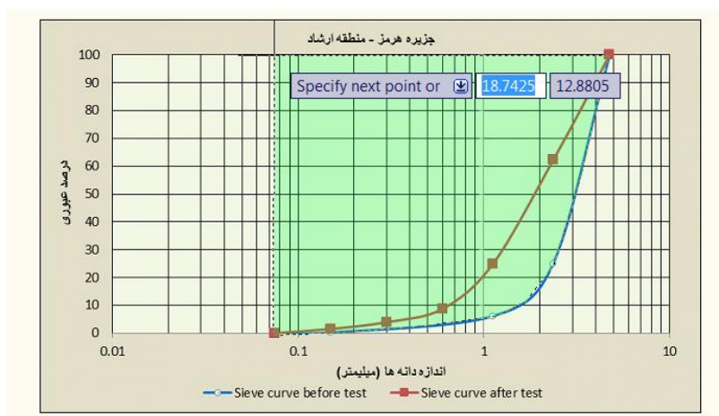
شکل ۹. نمایش محاسبه سطح بین نمودار دانه‌بندی اولیه و خط ۷۵ میکرون
