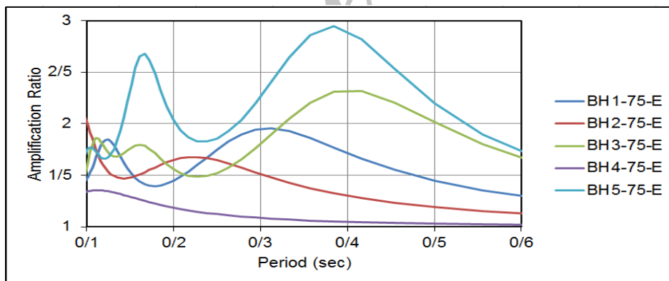
شکل ۱۲. طیف تقویت پروفیل‌های انتخابی با دوره بازگشت ۷۵ سال خروجی برنامه آرا
