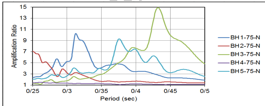
شکل ۱۵. طیف تقویت پروفیل‌های انتخابی با دوره بازگشت ۷۵ سال خروجی برنامه ترا
