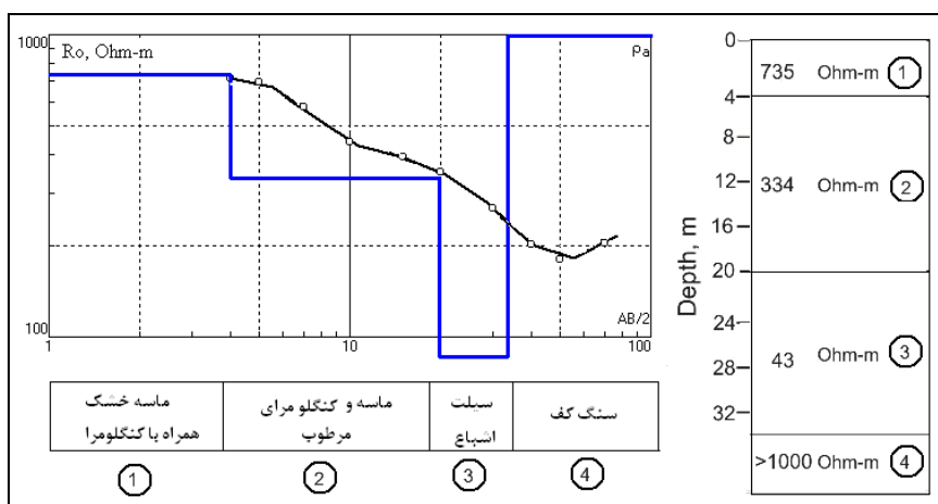
۵. نمودار چاهک الکتریکی و مدل ژئوالکتریکی مقطع زمین‌شناسی در محل پایه شرقی پیل
