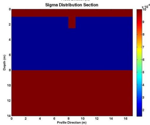
شکل ۸. مدل فیزیکی و هندسی زمین سه لایه‌ای شامل چندضلعی دوبعدی در قسمت پایین شکل و پاسخ سامانه GPR شبیه‌سازی شده متناظر با پروفیل مورد نظر در قسمت بالای شکل
