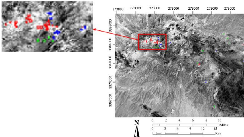
شکل ۷. مناطق آموزشی زون های دگرسانی مختلف (قرمز: آرژیلیک، سبز: فیلیک، آبی: پروپیلیتیک)
