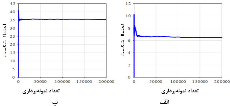
شکل ۹. بررسی هم‌گرایی احتمال شکست برای شرایط الف) استاتیکی، ب) شبه استاتیکی
