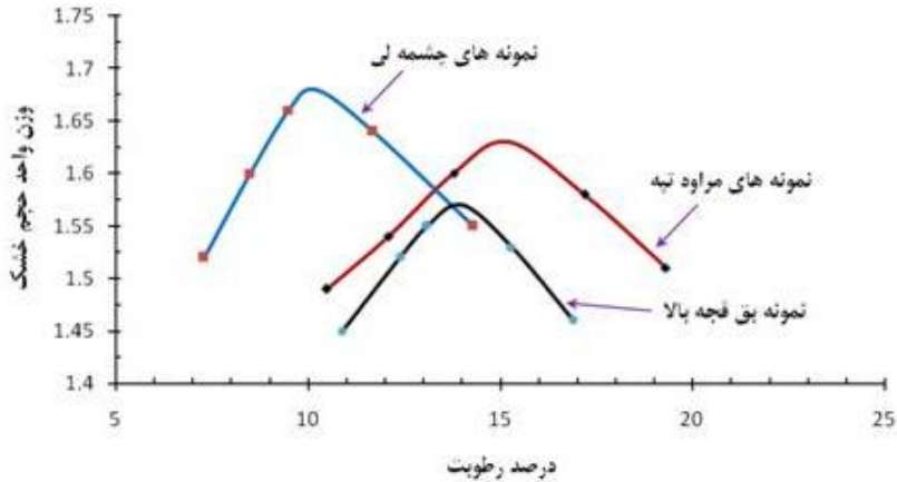
شکل ۴. منحنی‌های تراکم پروکتور استاندارد (معمولی)
