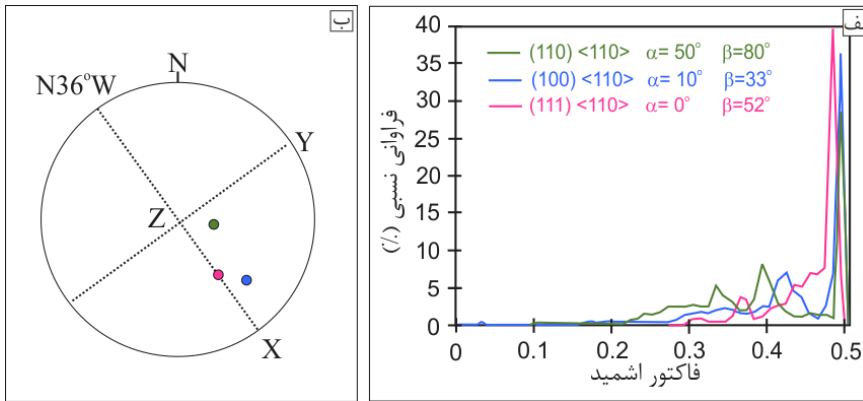
شکل ۶. نتایج تجزیه عامل اشمید، الف) منحنی‌های فراوانی عامل اشمید برای سه سیستم لغزشی موجود در بلورهای حالت، ب) موقعیت تنش‌های تراکمی مربوط به بیش‌ترین مقدار عامل اشمید برای هر سیستم لغزشی در استریوت
