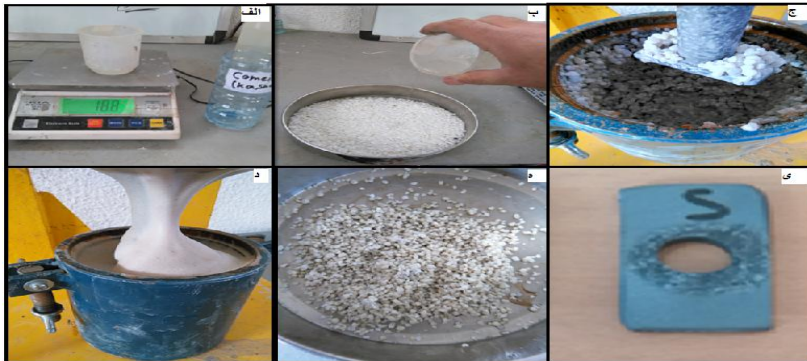
شکل ۱۲- مراحل انجام آزمایش تعیین ساینده‌گی مصالح فوم دار، الف) وزن کردن فوم، ب) افزودن فوم به مصالح، ج) آزمایش در حالت خیس شدگی، د) آزمایش در حالت مصرف زیاد فوم، ه) تصویر دانه‌ها بعد از آزمون، ی) تصویر ایمپلر بعد از آزمون
