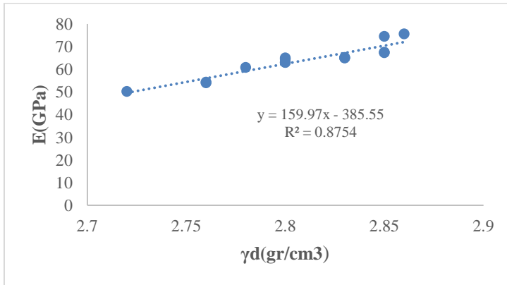
شکل ۱۰. رابطه بین مدول الاستیسیته با وزن واحد حجم خشک
