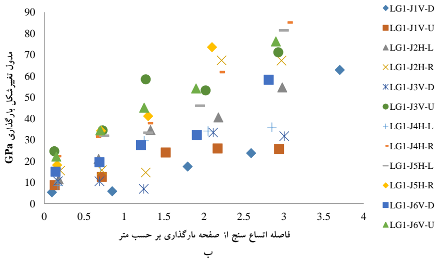
شکل ۵. تغییرات مدول بارگذاری در عمق الف) کوله راست سد بهشت‌آباد، ب) کوله چپ سد بهشت‌آباد
