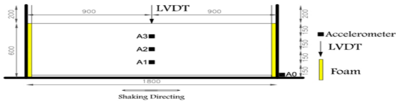
شکل ۲. شکل شماتیک نمونه‌های آزمایش همراه با ابزاربندی
