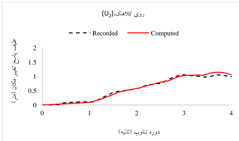
شکل ۱۱. طیف پاسخ تغییر مکان در محل اتصال پایه به کلاهک پل ملولند تحت زلزله ایمپریال ولی، ۱۹۷۹
