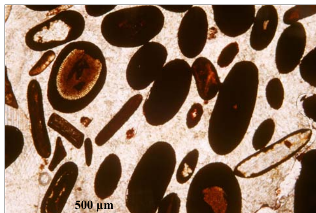
شکل ۴: اوولیدهای آهن دار با جورشدگی خوب. هسته اوولید از خرده‌های اسکلتی تشکیل شده است.
