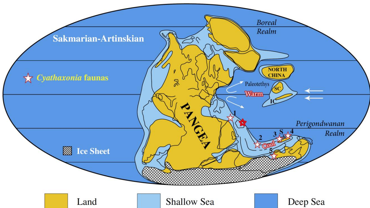
شکل ۴: پراکندگی زیست جغرافیایی مرجان‌های روگوزای سیاتاکسونیا در زمان پرمین پیشین (ساکمارین - آرتینسکین)؛ برگرفته از Wang et al., 2013. همراه با اندکی تغییرات (ستاره سرخ رنگ فون سیاتاکسونیای بلوک ایران مرکزی و ستاره‌های سفید رنگ حضور این فون در دیگر مناطق مشابه در کمربند سیمیرید را نشان می‌دهد).
