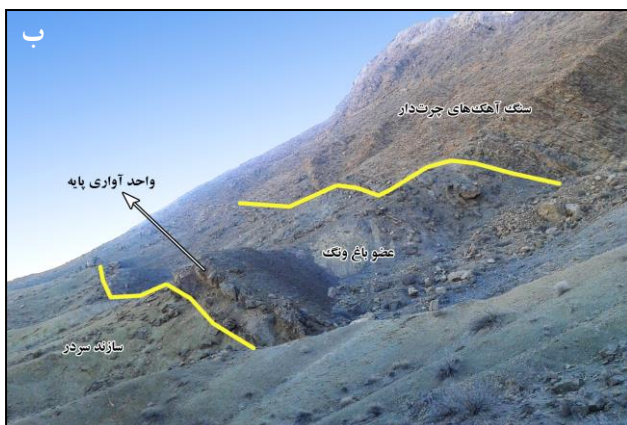
شکل ۲: عضو باغ‌ونگ سازند جمال و گذر آن با سازند سردر در زیر و سنگ آهک‌های چرت‌دار سازند جمال در بالا؛ الف) برش کوه باغ‌ونگ (جهت دید به
