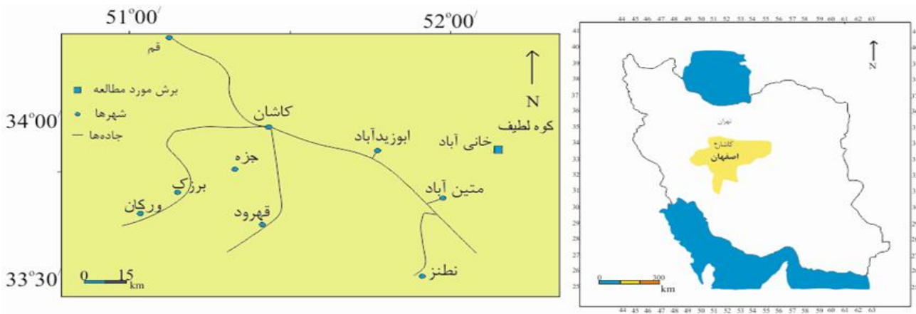
شکل ۱: راه‌های دسترسی به برش خانی‌آباد (برگرفته از بختیار، ۱۳۸۴؛ با اندکی تغییرات)
