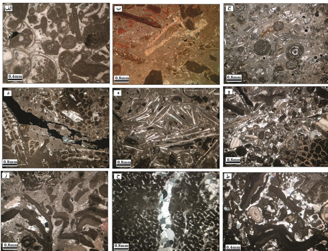
شکل ۳: ریزرخساره‌های موجود در نهشته‌های کریناته سازند قم در برش خانی‌آباد؛ الف) گریستون حاوی بیوکلاست و روزن‌داران کفزی، ب) وکستون بیوکلاست‌دار، ج) وکستون دارای روزن‌داران کفزی، د) وکستون حاوی بیوکلاست و بریوزوئر، ه) وکستون حاوی دوکفه‌ای، و) وکستون حاوی بیوکلاست، دوکفه‌ای و بریوزوئر، ز) وکستون - وکستون حاوی جلبک قرمز و روزن‌داران کفزی، ح) باندستون مرجانی، ط) گریستون حاوی جلبک قرمز و بیوکلاست.
