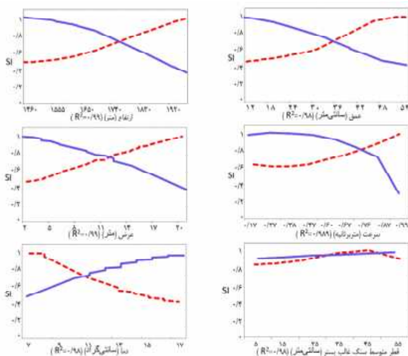
شکل ۲: نمودارهای رابطه مقادیر شاخص مطلوبیت و متغیرهای زیستگاهی (خط چین قرمز برای گروه < ۱۱ سانتی متر و خط ممتد آبی برای گروه > ۱۱ سانتی متر)
