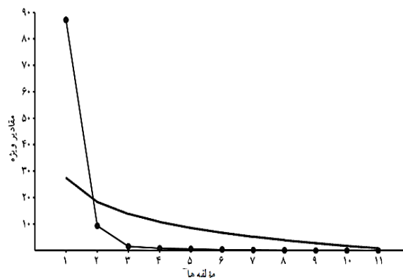
شکل ۲: نتایج Scree plot تحلیل مؤلفه‌های اصلی و نمایش نقطه برش جولیف (خط ممتد) که نشان‌دهنده مرز مؤلفه‌های اصلی (دایره‌ها) معنی‌دار است.
