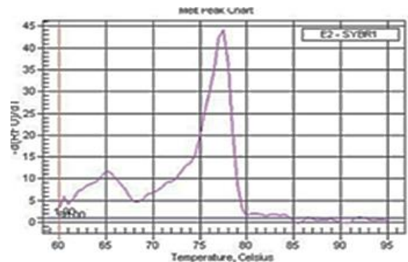
شکل ۲: منحنی ذوب ترسیم شده از غلظت‌های سریالی برای آغازگر Vtg
