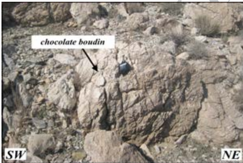
شکل ۶- توده‌ی کلسیتی بودین شده به فرم تخته شکلاتی که دو راستای کشش تقریباً عمود بر هم را نشان می‌دهد. یک راستا E 10° N که با راستاهای کشش در شکل ۵ هم‌خوانی دارد و دیگری راستای N 295° E که بر آن عمود است.
