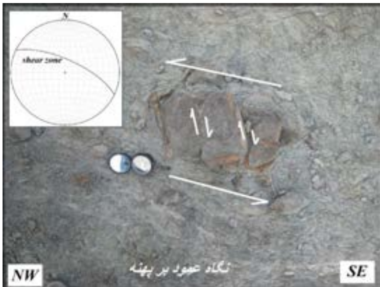
شکل ۷- بودین دومینو شکل که در یک پهنه‌ی برشی چپگرد شکل گرفته است. استریونت مربوط به پهنه‌ی برشی که این بودین در آن شکل گرفته است، در گوشه‌ی سمت چپ و بالای شکل آورده شده است.
