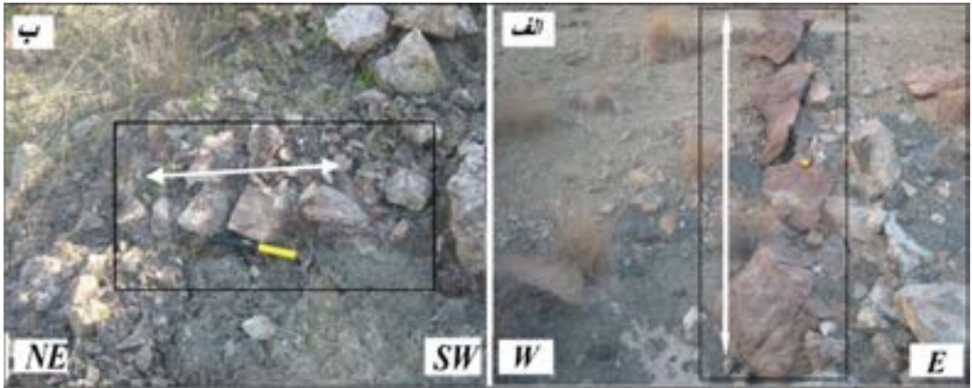
شکل ۵- بودین‌های مشاهده شده در منطقه که هر دو مورد تقریباً راستای کششی یکسانی را نشان می‌دهند. (الف) راستای کشیدگی E 10° N. (ب) راستای کشیدگی E 20° N.
