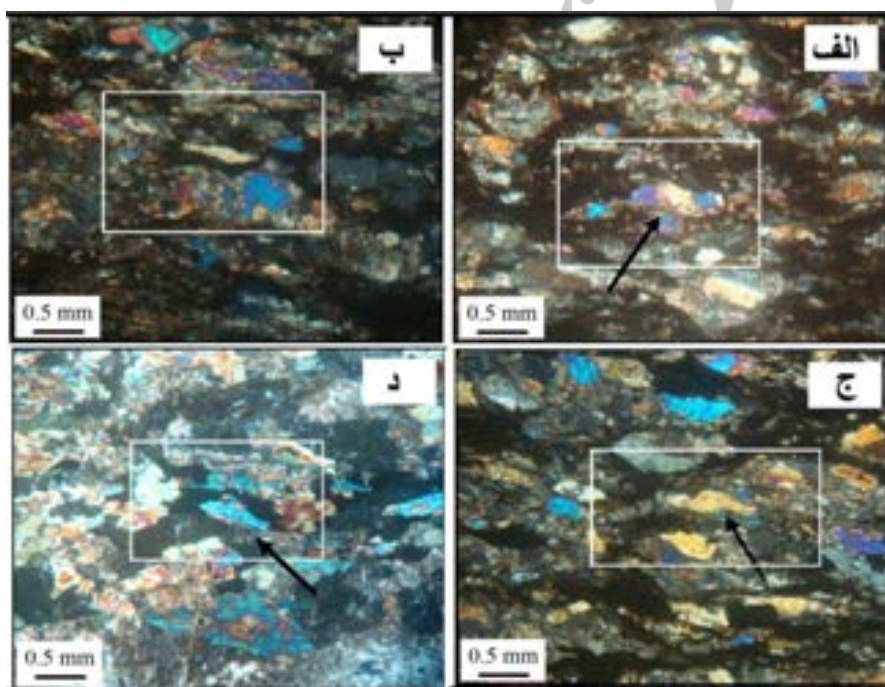
شکل ۱۱- مقاطع میکروسکوپی تهیه شده از میلونیت‌های منطقه؛ الف، ب، ج، د) با توجه به فرم پورفیروکلاست‌های میکا که در مقاطع دیده می‌شود، میکا ماهی‌ها نشان دهنده‌ی اعمال برش چپ‌گرد هستند.
