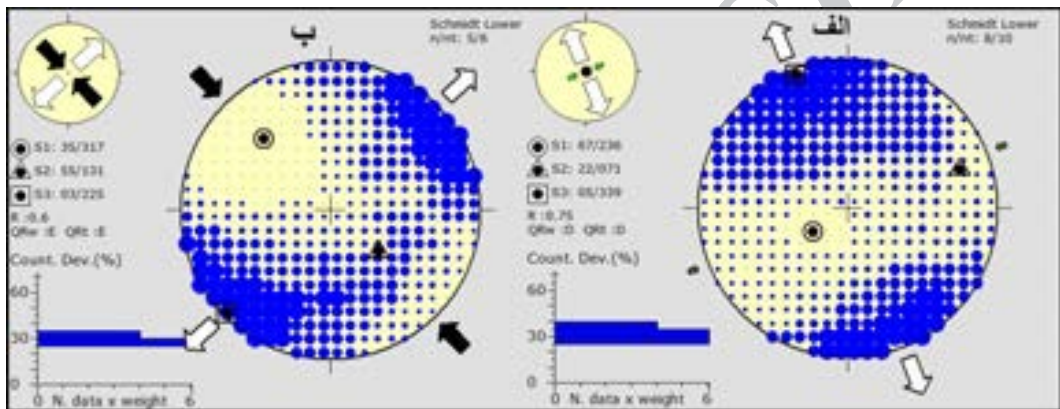
شکل ۴- تعیین جهت تنش دیرینه به روش برگشتی همراه با زاویه‌ی ناهمخوانی (محور افقی تعداد داده و محور عمودی زاویه‌ی ناهمخوانی)، موقعیت \sigma_1 ، \sigma_2 و \sigma_3 در هر استریوپلات به ترتیب با \blacksquare ، \blacksquare و \blacksquare مشخص شده‌است. الف- صفحات گسلی دارای مؤلفه‌ی امتدادی راست‌گرد، ب- صفحات گسلی دارای مؤلفه‌ی امتدادی چپ‌گرد.
