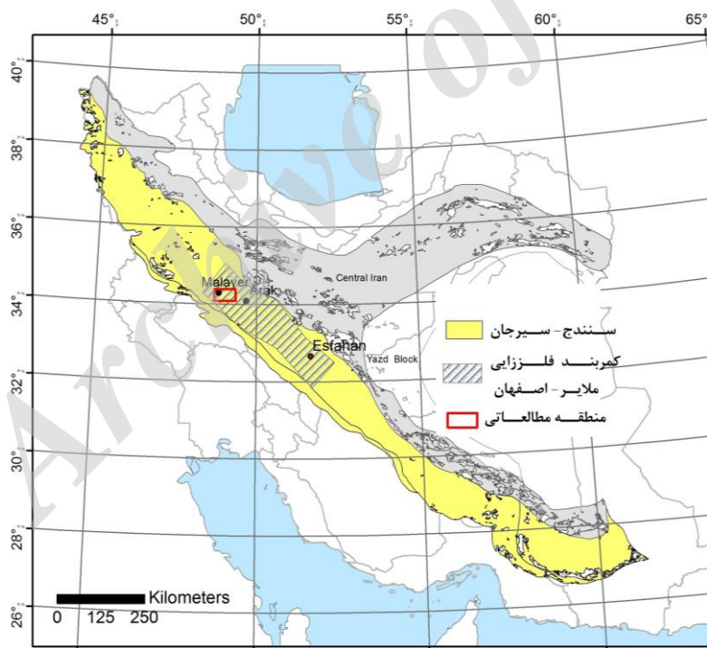
شکل ۱: بخشی از تقسیم‌بندی زون‌های ساختاری ایران (علوی، ۱۹۹۴) و موقعیت منطقه مطالعاتی درون کمریند فلززایی سرب و روی ملایر- اصفهان
