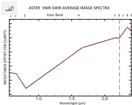
شکل ۱۲: الف) طیف میانگین تصویری واحد ماسه‌سنگی قاعده کرتاسه بازنویسی شده به محدوده باندهای VNIR_SWIR استر. ب) نمایی از واحد ماسه‌سنگی قاعده کرتاسه زیرین (Kc) بصورت افق سیاه رنگ در قاعده واحدهای کربناته کرتاسه زیرین (واحد Km, Kl).
