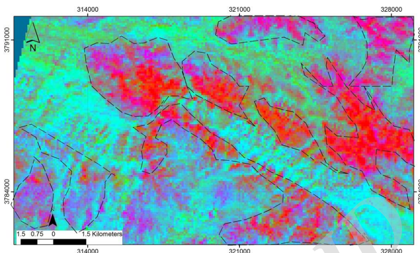
شکل ۶: تصویر Decorrelation-Stretch ترکیب رنگی (۱۰، ۱۲، ۱۴: RGB) استر منطقه مطالعاتی. در این تصویر ماسه سنگ‌ها و شیل‌ها - رسوبات آبرفتی همراه به ترتیب به رنگ قرمز و آبی تیره (خط چین سیاه رنگ) و کربنات‌ها به رنگ آبی فیروزه‌ای مشاهده می‌شوند.
